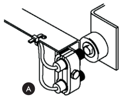
A Anbringung des Referenzsensors
